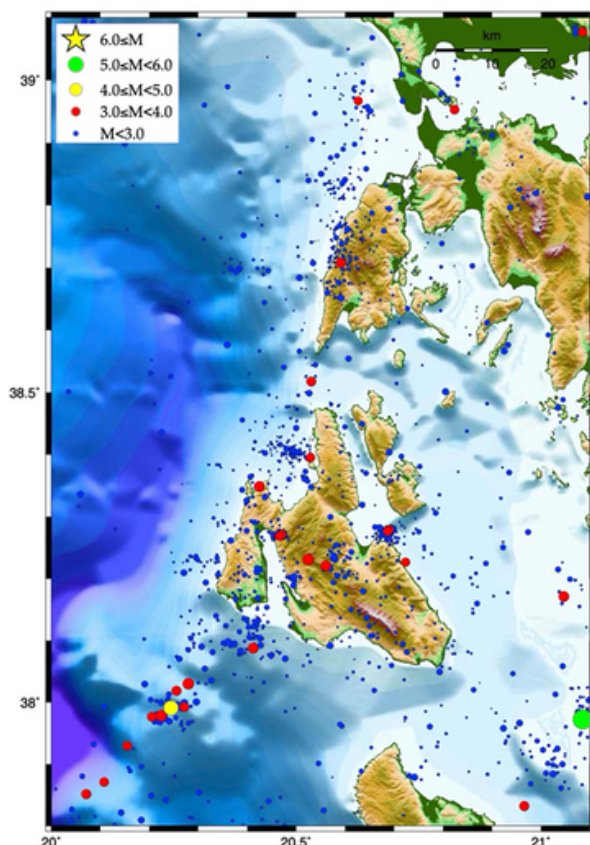
Σχ. 2. Κατανομή των epicέντρων των σεισμών που έγιναν στη διάρκεια Α εξαμήνου του 2025 στο χώρο των κεντρικών Ιονίων Νήσων.
