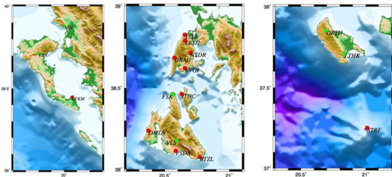
Σχ. 1. Χάρτες της περιοχής των Ιονίων νήσων στους οποίους φαίνεται το εγκατεστημένο δίκτυο σεισμολογικών σταθμών που λειτουργεί με τη συνεργασία της ΠΕΔ-IN και του ΑΠΘ (κόκκινα εξάγωνα). Με πράσινα εξάγωνα παριστάνονται σεισμολογικοί σταθμοί άλλων δικτύων στην περιοχή.
