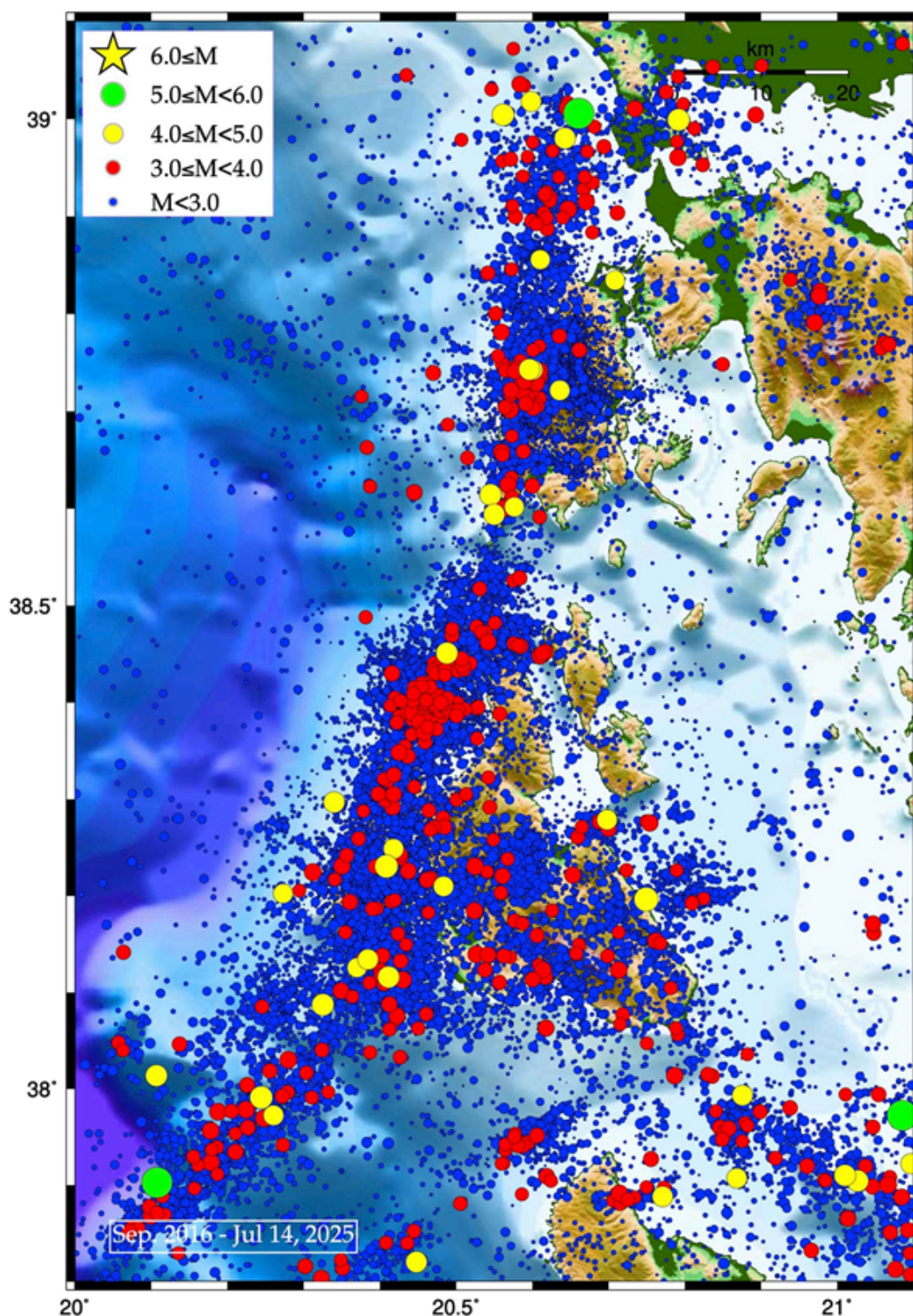
Σχ. 7. Επίκεντρα των σεισμών που έχουν γίνει στο χώρο των κεντρικών Ιονίων νήσων στο χρονικό διάστημα Σεπτέμβριος 2016 – Ιούνιος 2025.
