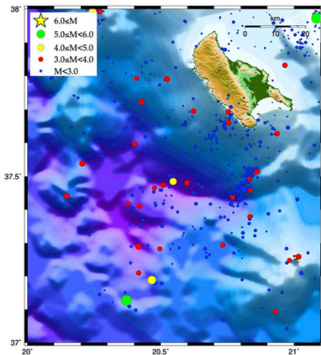
Σχ. 5. Κατανομή των epicέντρων των σεισμών που έγιναν στη διάρκεια του Α εξαμήνου του 2025 στην ευρύτερη περιοχή της Ζακύνθου.
