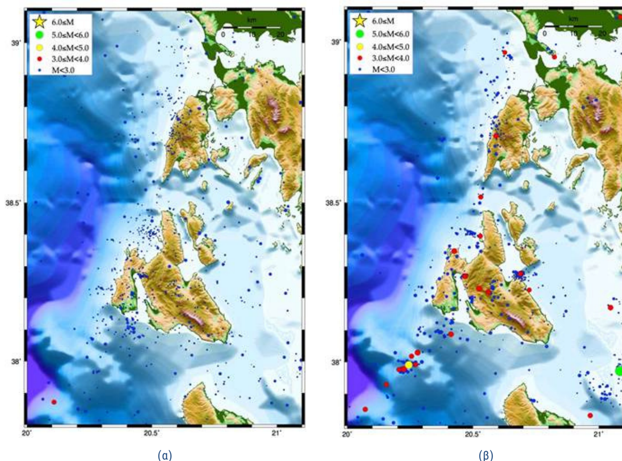
Σχ. 3. Κατανομή των επικέντρων των σεισμών στα κεντρικά Ιόνια Νησιά: (α) Σεισμοί οι οποίοι αναλύθηκαν μόνο από την ομάδα παρακολούθησης της σεισμικής δραστηριότητας στην περιοχή στο πλαίσιο της παρούσας προγραμματικής σύμβασης. (β) Σεισμοί οι οποίοι αναλύθηκαν και από τους σεισμολογικούς φορείς της Ελλάδας και δημοσιεύονται στα Δελτία τους.
