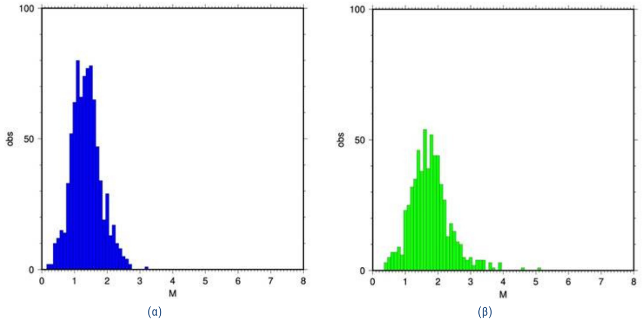
Σχ. 4. Ιστογράμματα της κατανομής των μεγεθών των σεισμών στα κεντρικά Ιόνια νησιά. (α) Σεισμοί που αναλύθηκαν μόνο από την ομάδα εργασίας στο πλαίσιο της παρούσας προγραμματικής σύμβασης. (β) Σεισμοί που αναλύθηκαν και από τους σεισμολογικούς φορείς της Ελλάδας.
