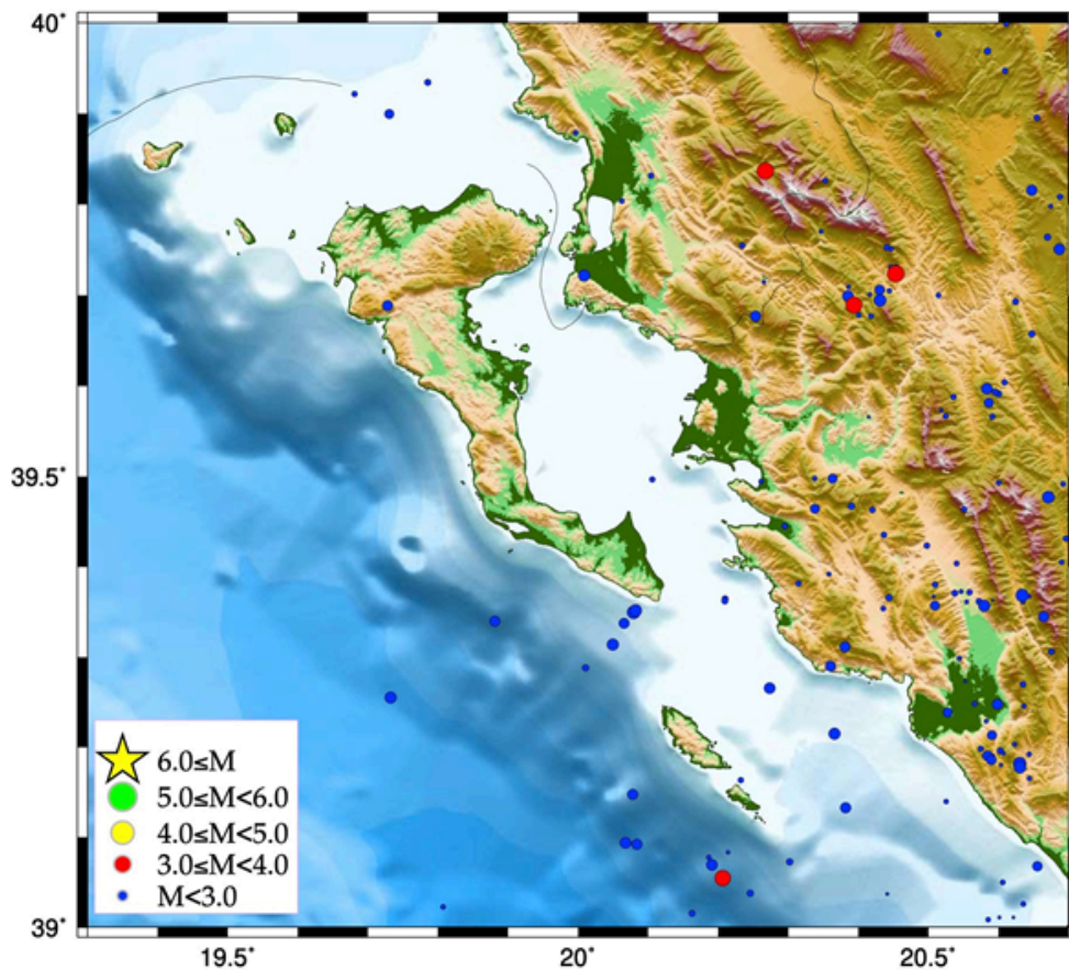
Σχ. 6. Τα επίκεντρα των σεισμών που έγιναν στη διάρκεια του Α εξαμήνου του 2025 στο Βόρειο Ιόνιο.
